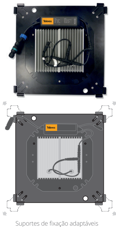
Suportes de fixação para luminária "Villa"
