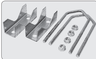
Art.nr: 531 00 04 Mastbygel MB-50P, med klammer. E-nr: 60 005 77
