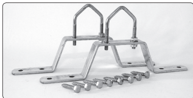
Art.nr: 522 21 01 Väggfäste VF-210, 7,5 cm från vägg. För rör 30–50 mm. Levereras i par. E-nr: 60 611 40
