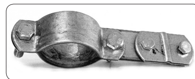
Art.nr: 550 01 64 Rörklove RKJ-50 för HF-jordning av maströr passar 50 mm rör. E-nr: 60 611 35
