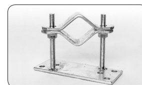
Art.nr: 527 75 05 RK-50/76 (Enkel) höger justerbar 0-75 mm från vägg rör 50-76 mm. E-nr: 60 720 17
