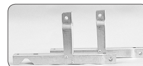
Art.nr: 523 51 01 Skorstensfäste SF-205-1. Ett par inklusive 5 m, rör 30-50 mm. E-nr: 60 611 15
