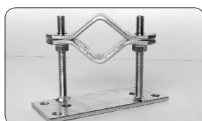
Art.nr: 527 75 06 RK-50/76 (Enkel) vänster justerbar 0-75 mm från vägg rör 50-76 mm. E-nr: 60 720 18
