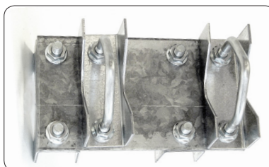
Art.nr: 525 40 01 Mastadapter rör 32–50 mm, för att montera extra rör parallellt med befintligt. E-nr: 60 611 39
