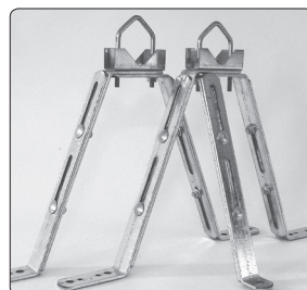
Art.nr: 522 34 05 Väggfäste VF-2550P par, 25-45 cm från vägg, för rör 30-50 mm. E-nr: 60 611 42
