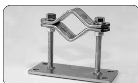
Art.nr: 527 75 07 RK-50/76 (Enkel) justerbar 0-75 mm från vägg rör 50-76 mm. E-nr: 60 611 23
